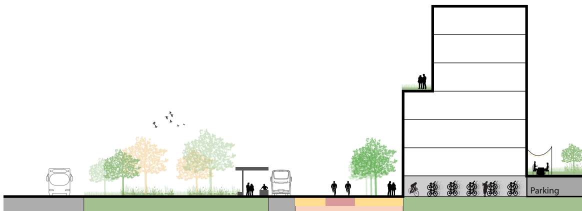
▲ Doorsnede 2 (exclusief sportzaal). Voorbeeld inrichting plein, inpassing busstation en relatie bebouwing.
